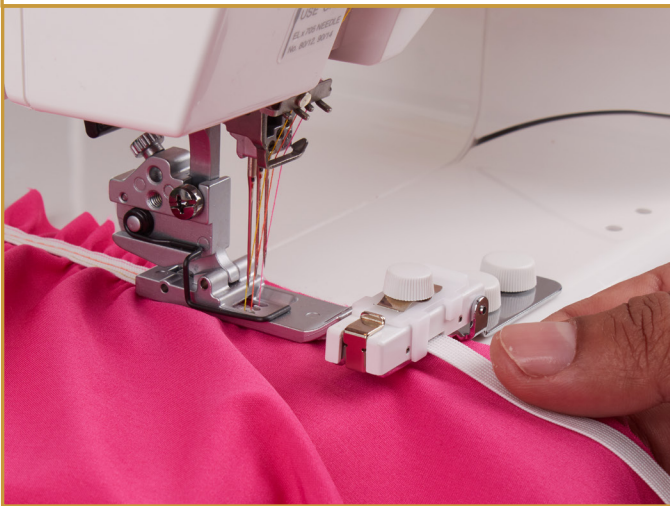
APARELHO PARA APLICAÇÃO DE ELÁSTICO
